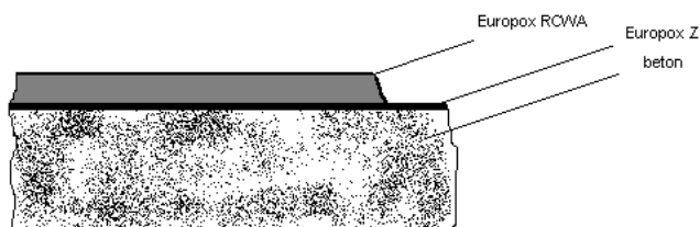
Rys. Warstwy systemu RCWA
